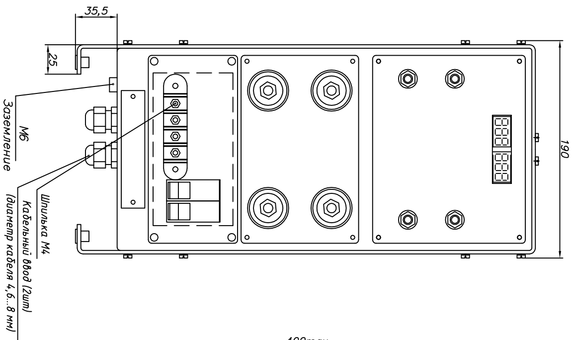
Зарядное устройство ЗУ 20 Габаритный чертеж
